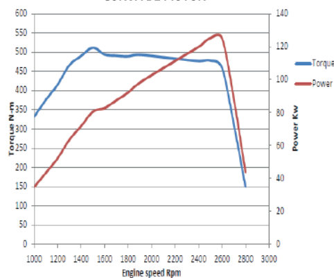
CURVA DE MOTOR
