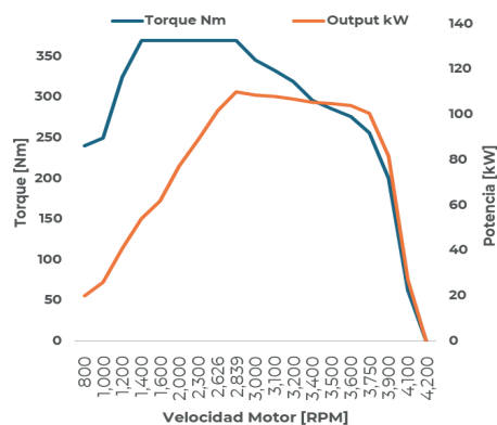
CURVA DE MOTOR 4P10 WAT 4 110 kW -- 2,839 RPM 370 Nm -- 1,400 - 2,839 RPM
